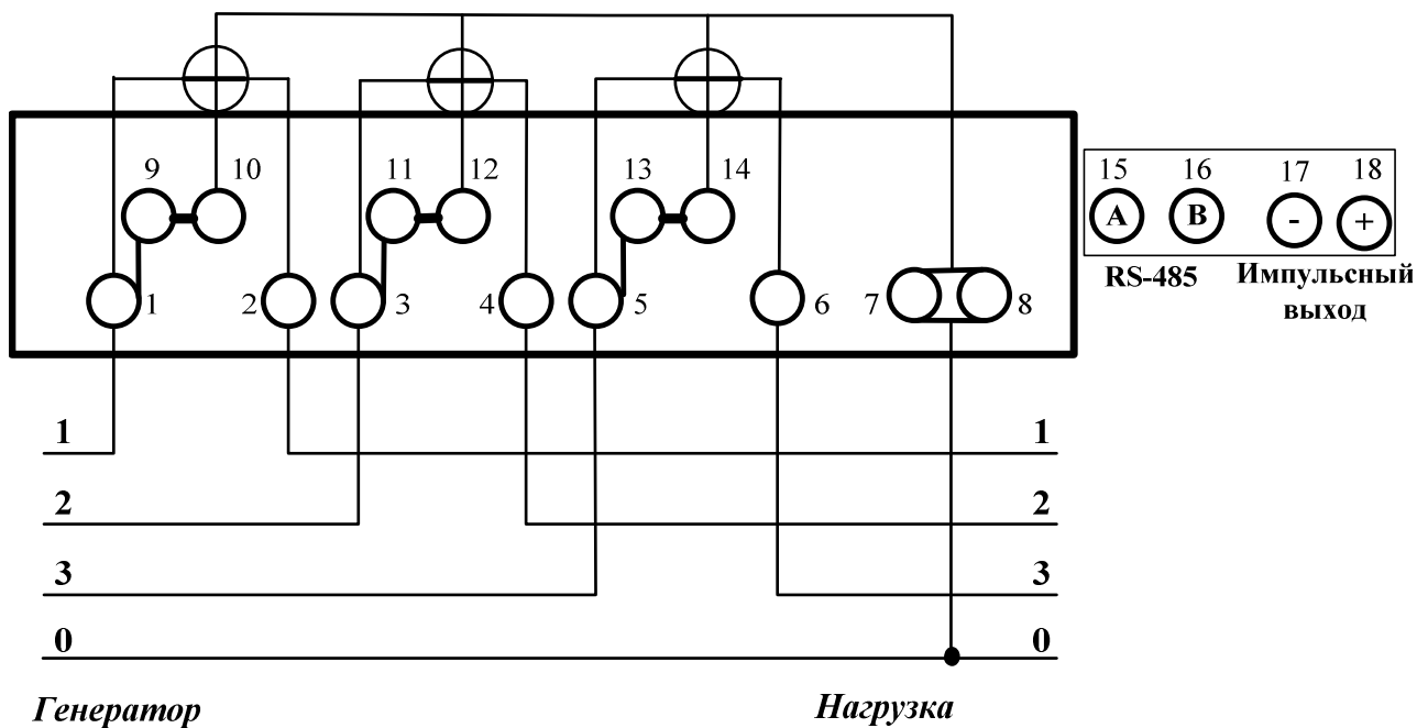
Рисунок Б.1 – Схема непосредственного подключения счётчика
