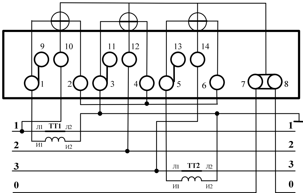
Рисунок Б.3 – Схема подключения счётчика с помощью двух трансформаторов тока
