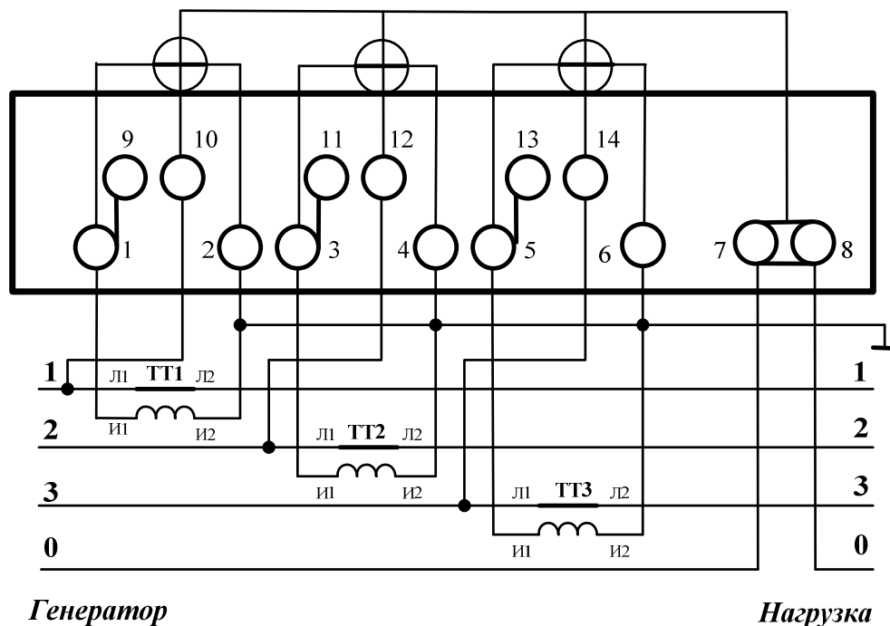
Рисунок Б.2 – Схема подключения счётчика с помощью трёх трансформаторов тока
