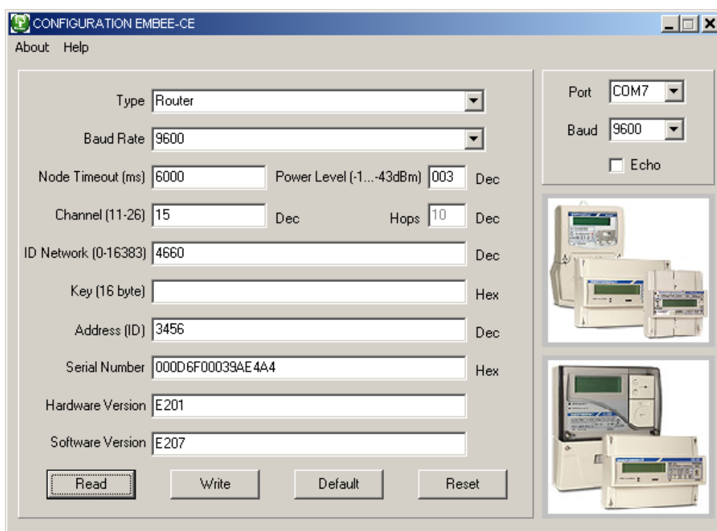
Рисунок 44 – Config-EMBee-CE конфигурирования встроенного радиомодуля
