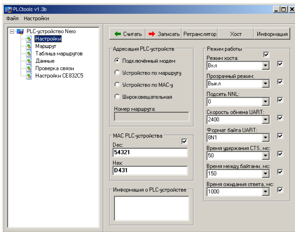
Рисунок 49 – Настройки PLC-модема
