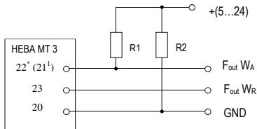
Рисунок 2.1 Подключение испытательных выходов счетчиков HEBA MT3
