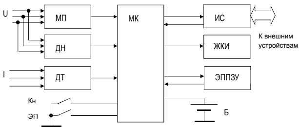
Рисунок 1 Функциональная схема счётчика.
